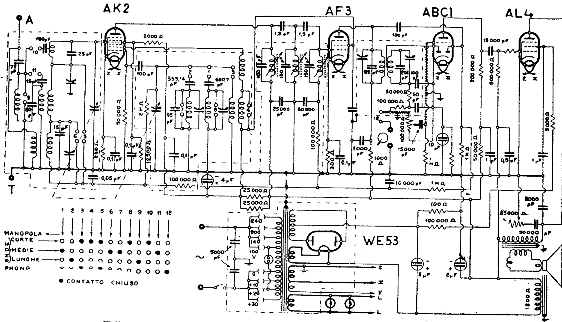
F.I.M.I. - MODD. PHONOLA « 850 » - « 851 » - « 853 »
